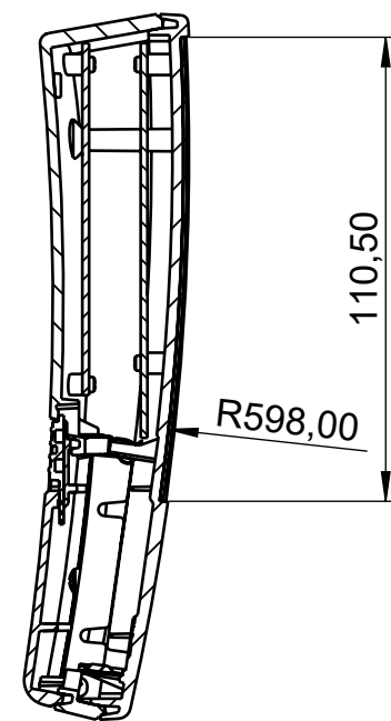
Schnitt C-C
