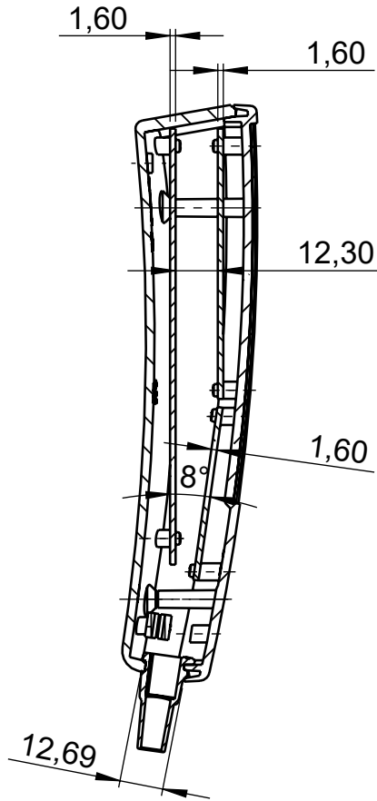
Schnitt B-B
