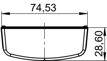
Schnitt C-C
