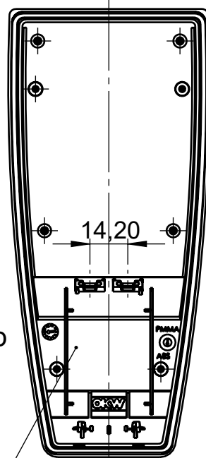
Oberteil Innenansicht Top part inside view
