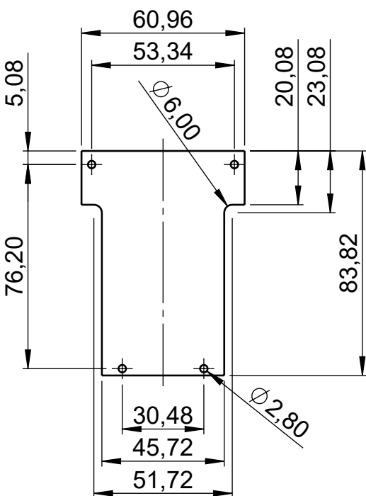
Platine für Unterteil mit Batteriefach PCB for base part with battery compartment
