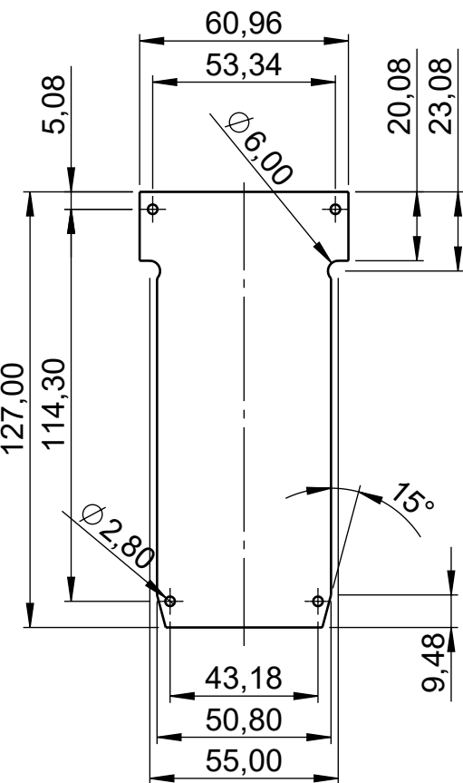
Platine für Unterteil ohne Batteriefach PCB for base part with battery compartment
