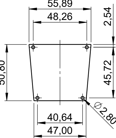
Platine für Oberteil ohne Batteriefach PCB for top part without battery compartment
