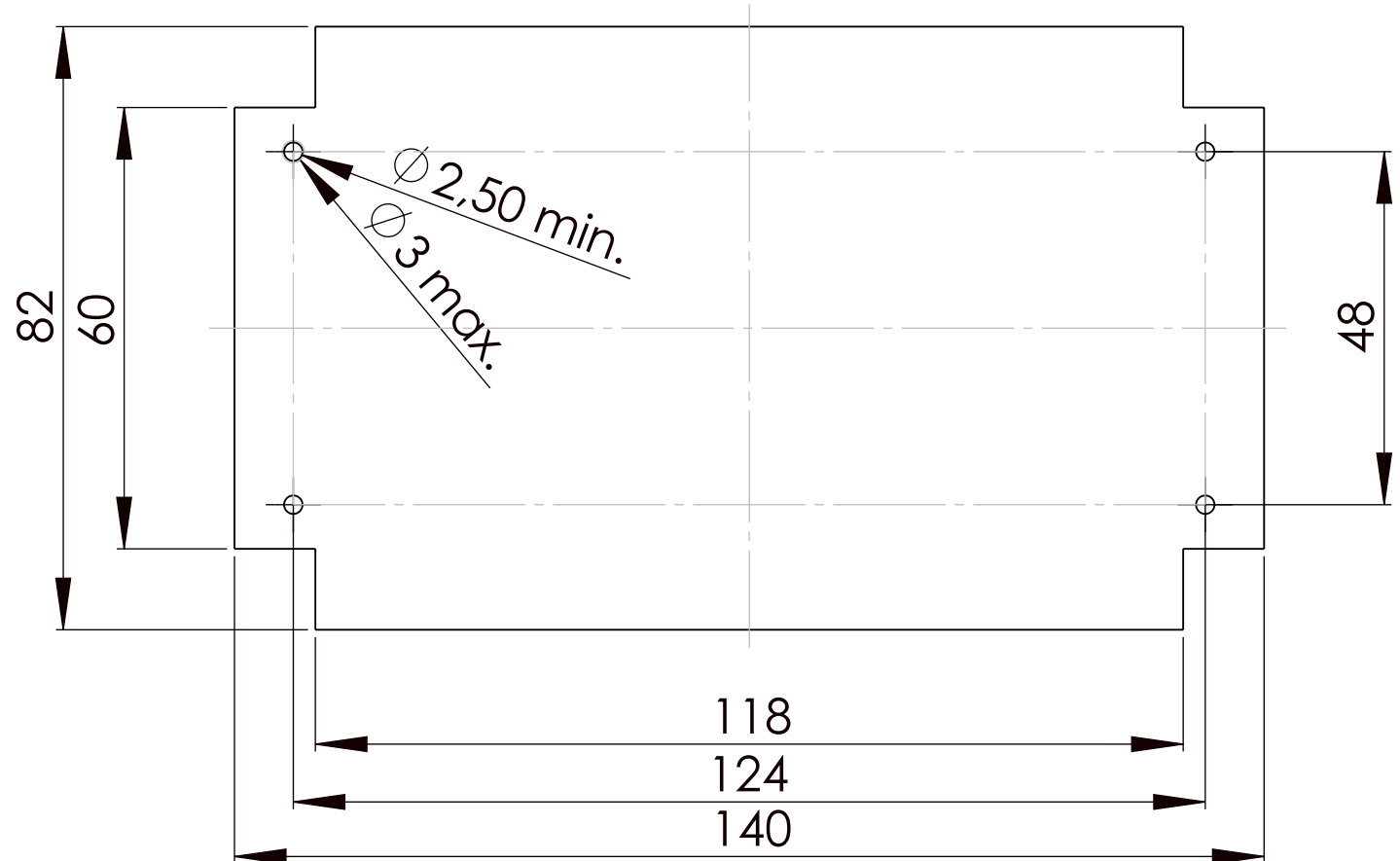
Platine UT P C B
