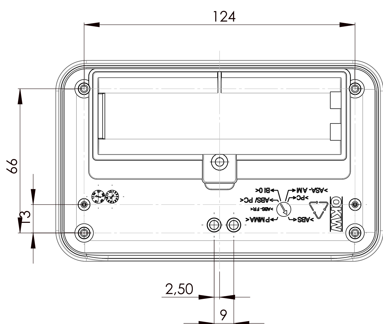
Unterteil mit Batteriefach 4x1,5V Bottom-Part with battery-compartment 4x1,5V
