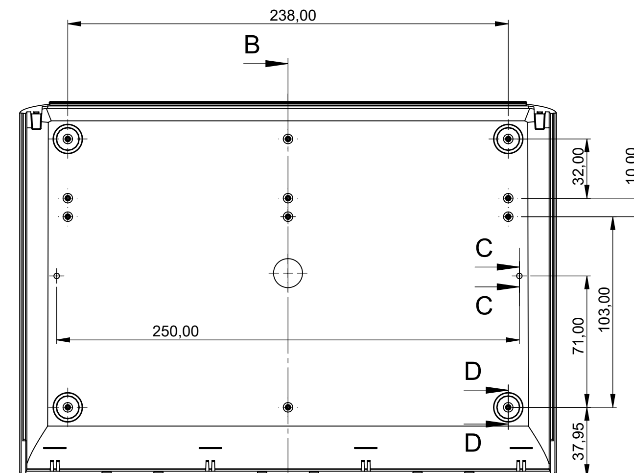
Unterteil- Innenansicht BASE, REAL INSIDE- VIEW
