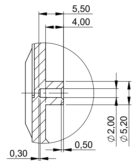
Detail Y
