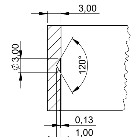
Schnitt C-C (2:1)
